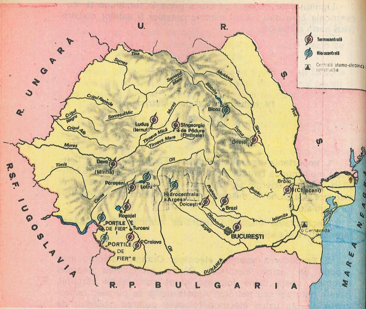
Principalele termocentrale și hidrocentrale
