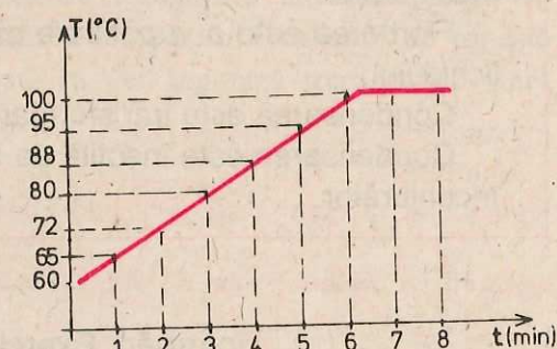
Fig. 3.2.19. Diagrama fierberii apei.
