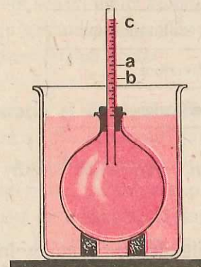
Fig. 3.2.6. Dilatația lichidelor.
