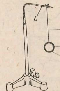
Fig. 3.3.7. Pendulul electric: (1) foiță de staniol, (2) foia de plută, (3) fir de mătase, (4) suport de sticlă.
