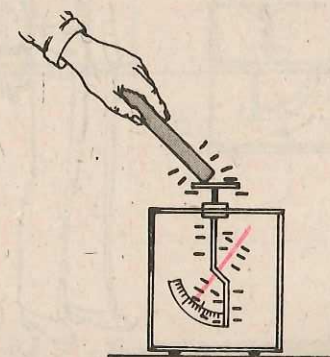
Fig. 3.3.11. Încărcarea electroscopului, prin contact, cu sarcini negative.
