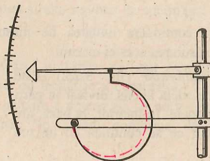
Fig. 3.2.4. Termometru metalic.
