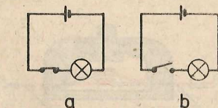
Fig. 3.3.34. Schema unui circuit electric simplu: a) circuit închis conținând generatorul, întrerupătorul, un bec și conductoare de legătură; b) același circuit, deschis.
