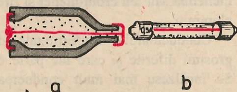
Fig. 3.3.42. Siguranțe fuzibile: a) siguranță folosită în instalația electrică; b) siguranță folosită la aparatele electrice.
