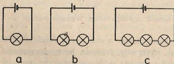
Fig. 3.3.35. Legarea becurilor în serie: a) fiecare bec legat pe rând, la baterie, emite o lumină la fel de intensă; b) două becuri legate în serie luminează mai slab; c) trei becuri legate în serie luminează foarte slab.
