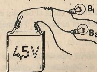
Fig. 3.3.40. Pentru exercițiul 10.
