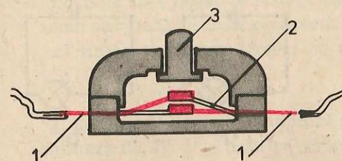
Fig. 3.3.30. Înterupător de sonerie.
