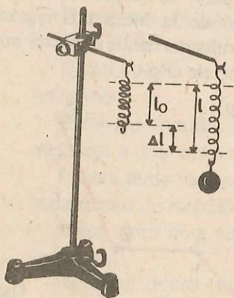
Fig. 3.1.17. Deformarea elastică a unui resort.
