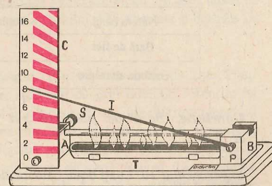
Fig. 3.2.7. Piometrul cu cadran.
