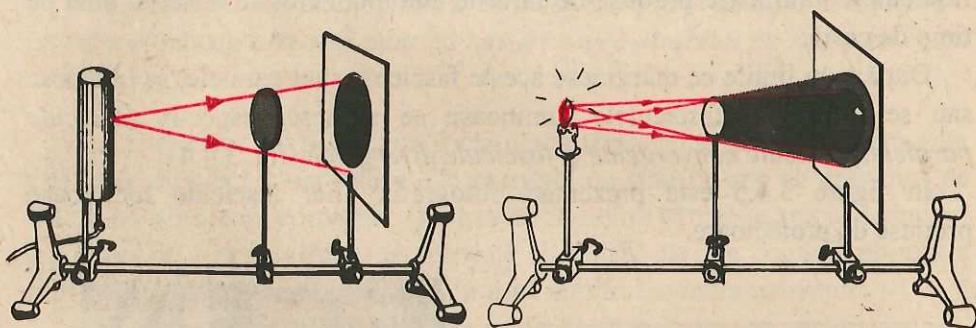
Fig. 3.4.6. Montaj experimental pentru observarea umbrei.
