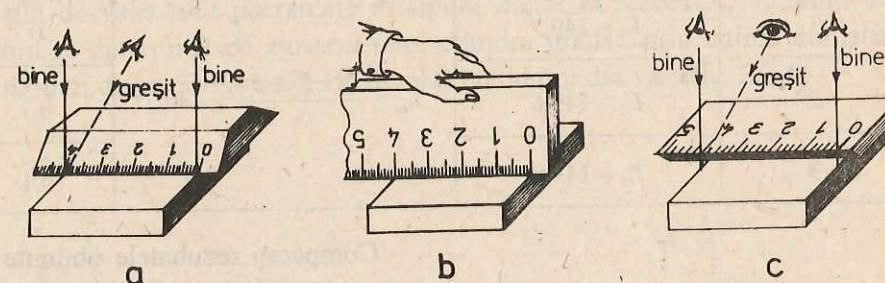
Fig. 2.2.3. Cum trebuie făcută citirea în cazul unei măsurări cu rigla.
