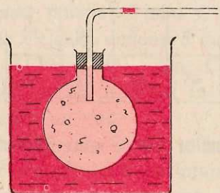
Fig. 3.2.5 Dilatația gazelor.
