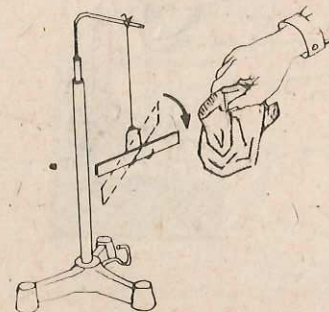
Fig. 3.3.6. Banda de celuloid și țesătura electrizate simultan prin frecarea lor se atrag reciproc.
