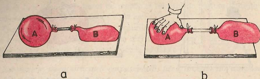
Fig. 2.1.7. Aerul are volumul vasului în care se află.
