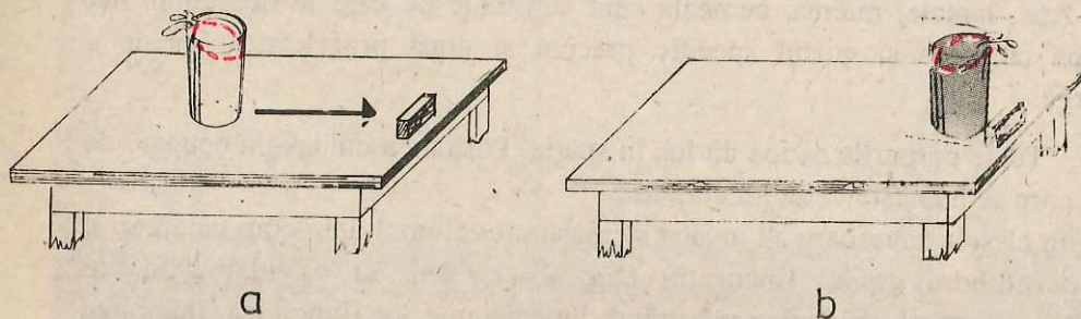
Fig. 2.1.2. a) Paharul plin cu apă este adus brusc în stare de mișcare; b) paharul plin cu apă este oprit brusc.
