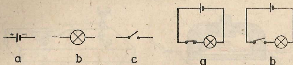
Fig. 3.3.33. Semne convenționale pentru elemente de circuit: a) generator; b) bec; c) întrerupător.
