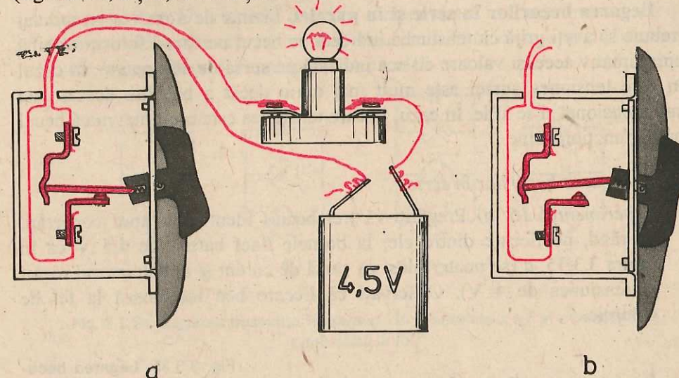
Fig. 3.3.32. Înterupător de lumină: a) poziție închis; b) poziție deschis.
