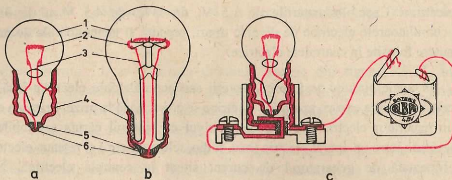
Fig. 3.3.29. Schema unui bec: a) bec de lanternă; b) bec folosit la iluminat; c) trecerea curentului electric prin conductoare, filament și baterie.
