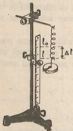
Fig. 2.3.1. Un corp suspendat de un resort determină alungirea resortului.
