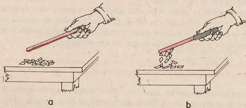
Fig. 3.3.3. a) Vergea de aluminiu ținută în mână și frecată cu țesătura de lână nu atrage bucățele de hârtie; b) vergea de aluminiu, prevăzută cu mâner izolator, frecată cu țesătura de lână, atrage corpuri ușoare.
