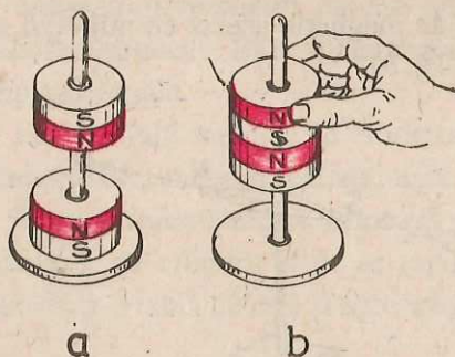
Fig. 3.3.20. Interacțiuni magnetice: a) doi magneti apropiați unul față de altul cu polii de același nume se resping reciproc; b) magnetii se atrag reciproc dacă sunt apropiați cu polii de nume diferite.
