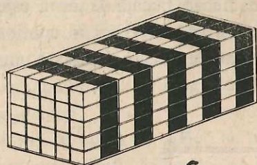
Fig. 3.3.22. Un magnet poate fi considerat ca fiind constituit dintr-un număr foarte mare de magneți mici.
