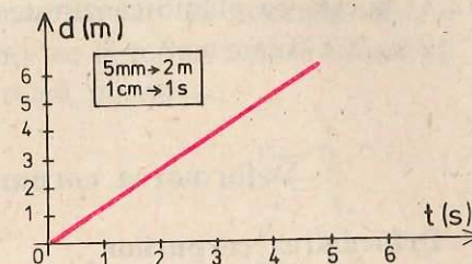
Fig. 3.1.15. Grafic pentru problema 7.
