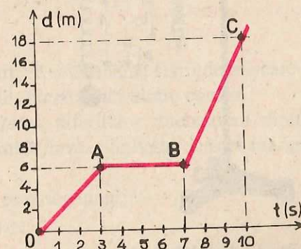
Fig. 3.1.16. Grafic pentru problema 8.
