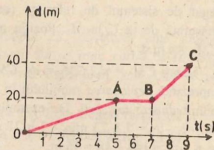
Fig. 3.1.9. Graficul unei mișcări.
