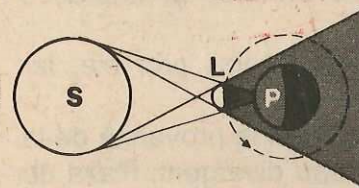
Fig. 3.4.8. Formarea eclipsei de Soare.
