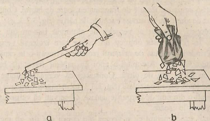
Fig. 3.3.2. a) În urma frecării cu țesătura de lână, celuloidul atrage bucățele de hârtie; b) în urma frecării cu banda de celuloid, țesătura de lână atrage bucățele de hârtie.
