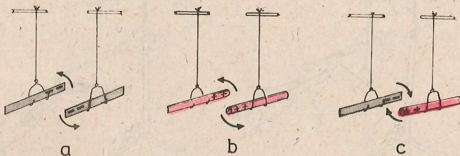
Fig. 3.3.5. a) Două benzi de celuloid electrizate cu sarcini negative se resping reciproc; b) două vergele de sticlă încărcate cu sarcini pozitive se resping reciproc; c) celuloidul electrizat cu sarcini negative și sticla electrizată cu sarcini pozitive se atrag reciproc.
