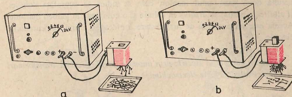
Fig. 3.3.48. a) Bobina parcursă de curent electric se comportă ca un magnet; b) bobină cu miez de fier.
