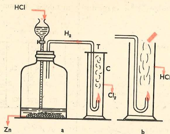
Fig. 2.7. Instalație pentru arderea hidrogenului în clor
