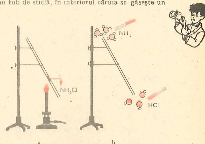
Fig. 4.13. Instalație pentru demonstrarea descompunerii termice a clorurii de amoniu
