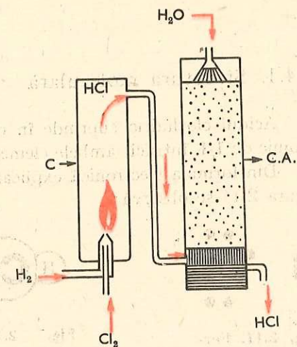
Fig. 2.13. Instalație industrială pentru obținerea acidului clorhidric prin sinteză
