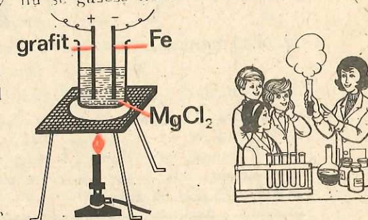
Fig. 8.3. Obținerea magneziului prin electroliza topiturii de clorură de magneziu
