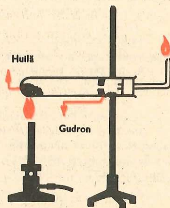
Fig. 5.12. Obținerea cocsului
