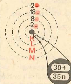
Fig. 11.21. Structura atomului de zinc (Izotopul ^{65}_{30}\text{Zn} )
