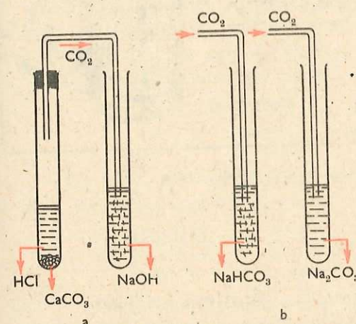
Fig. 7.7. Obținerea carbonaților acid și neutru de sodiu
