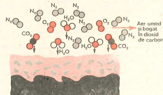
Fig. 11.3. Ruginirea fierului
