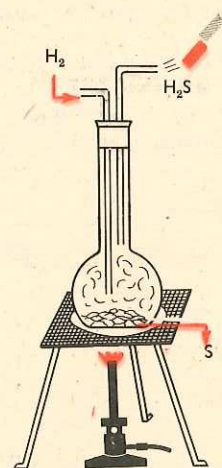
Fig. 3.9. Arderea hidrogenului în vapori de sulf
