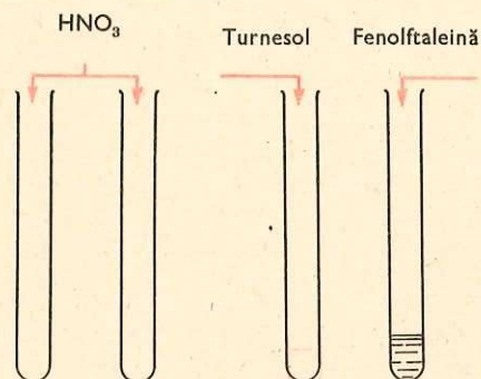
Fig. 4.20. Acțiunea acidului azotic asupra indicatorilor
