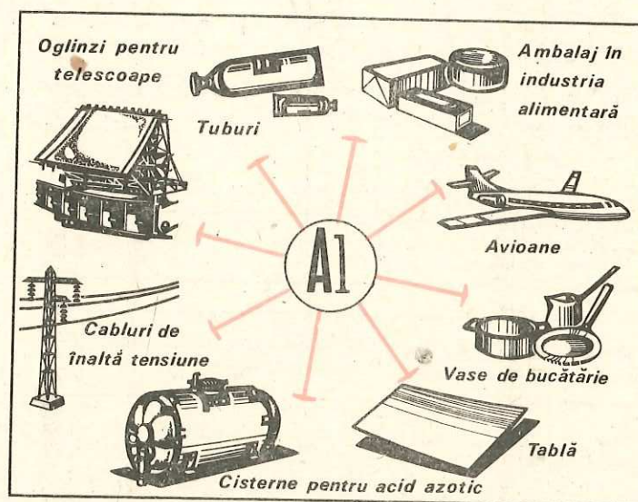
Fig. 9.5. Utilizările aluminului
