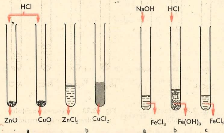
Fig. 2.21. Obținerea hidroxidului de fier (III) și acțiunea acidului clorhidric asupra acestuia
