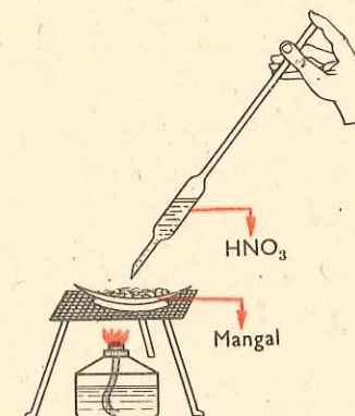
Fig. 4.24. Acțiunea acidului azotic asupra mangelului
