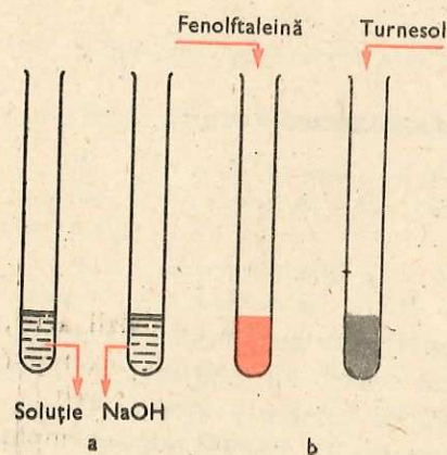
Fig. 7.4. Acțiunea hidroxidului de sodiu asupra indicatorilor
