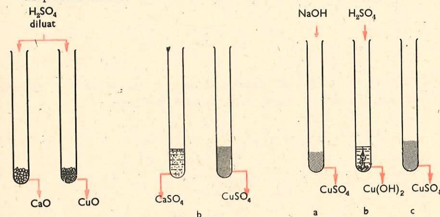
Fig. 3.18. Acțiunea acidului sulfuric asupra oxizilor metalici
