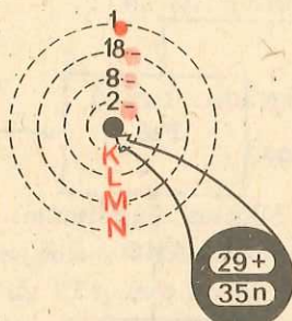
Fig. 11.16. Structura atomului de cupru (Izotopul ^{64}_{29}\text{Cu} )
