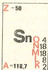
Fig. 10.1. Căsuța staniului în sistemul periodic
