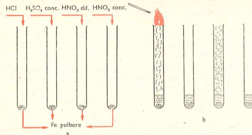
Fig. 11.7. Acțiunea acizilor asupra fierului
