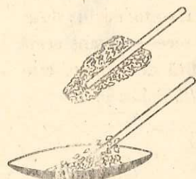
Fig. 3.6. Electrizarea sulfului prin frecare
