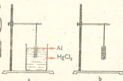
Fig. 9.8. Oxidarea aluminiului în aer, la rece
