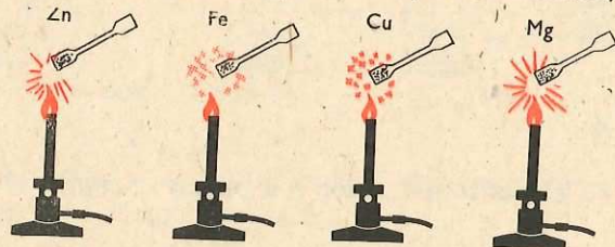
Fig. 6.10. Arderea metalelor în aer
