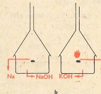
Fig. 6.12. Descompunerea apei de către potasiu și sodiu
