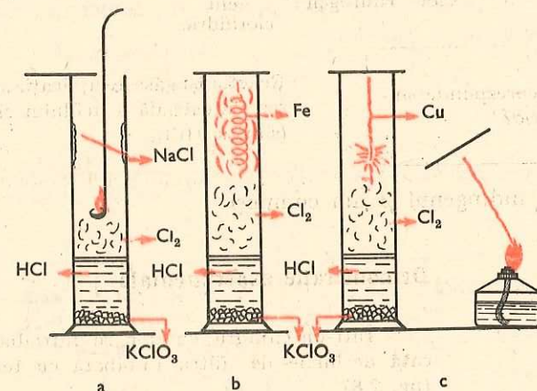
Fig. 2.10. Arderile metalelor în clor
