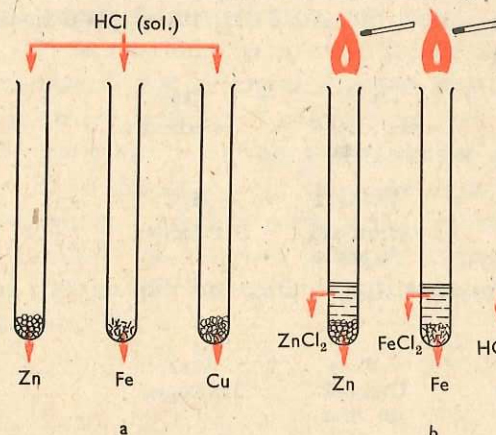
Fig. 6.13. Acțiunea acizilor asupra metalelor
