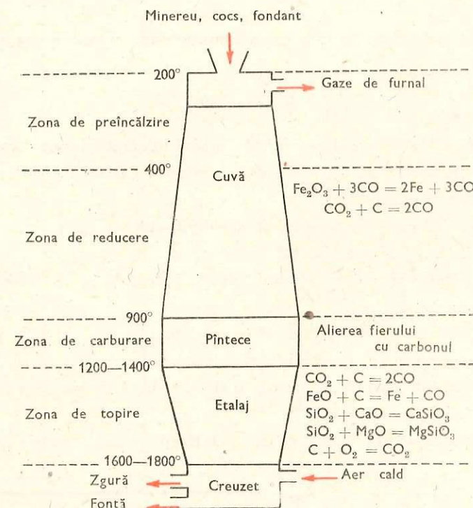
Fig. 11.10. Procesele fizico-chimice din furnal
