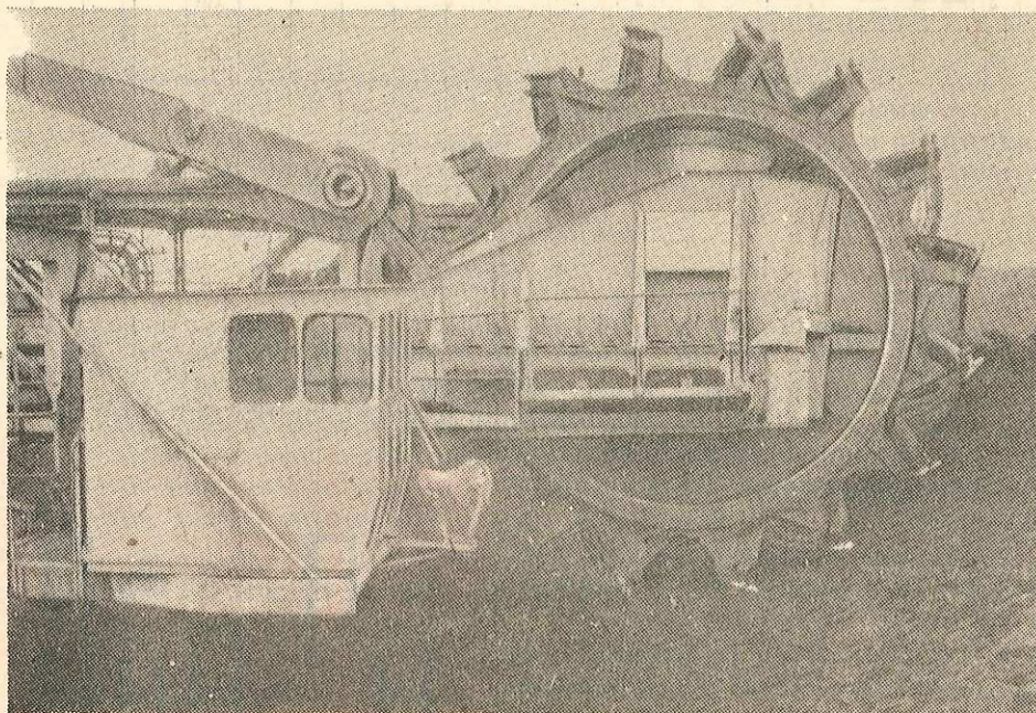
Exploatarea cărbunelui la zi la Întreprinderea Minieră Rovinari.
