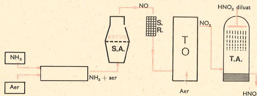
Fig. 4.17. Obținerea industrială a acidului azotic
