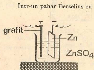
Fig. 11.24. Electroliza soluției de sulfat de zinc
