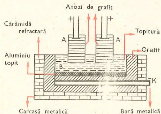
Fig. 9.4. Instalația pentru electroliza oxidului de aluminiu
