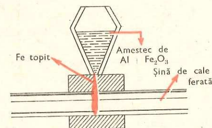
Fig. 9.10. Sudarea șinelor prin aluminotermie
