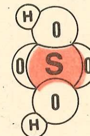
Fig. 3.12. Modelul moleculei de acid sulfuric
