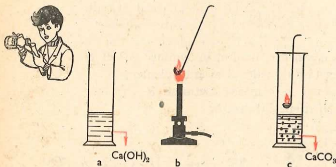
Fig. 5.9. Arderea cărbunelui și recunoașterea dioxidului de carbon rezultat
