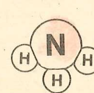
Fig. 4.6. Modelul molecular al amoniacului
