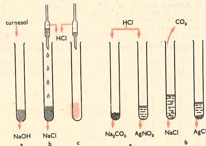
Fig. 2.23. Acțiunea acidului clorhidric asupra sărurilor
