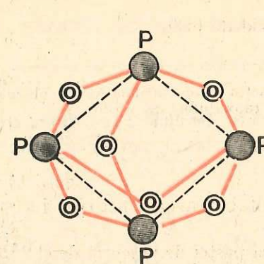
Fig. 4.33. Molecula trioxidului de fosfor \text{P}_4\text{O}_6
