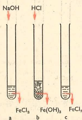
Fig. 2.21. Obținerea hidroxidului de fier (III) și acțiunea acidului clorhidric asupra acestuia
