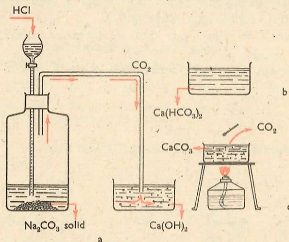
Fig. 8.13. Transformarea carbonatului neutru de calciu în carbonat acid de calciu și invers
