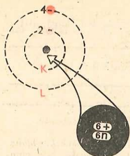
Fig. 5.3. Structura atomului de carbon (Izotopul ^{12}\text{C} )
