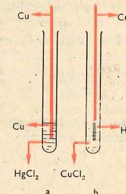
Fig. 6.14. Reacția dintre cupru și clorură de mercur
