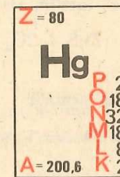
Fig. 11.22. Căsuța mercurului în sistemul periodic
