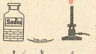
Fig. 7.3. Topirea sodiului
