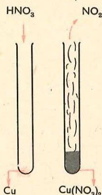
Fig. 4.21. Acțiunea acidului azotic asupra cuprului
