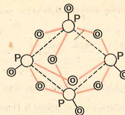
Fig. 4.34. Molecula pentaoxidului de fosfor \text{P}_4\text{O}_{10}
