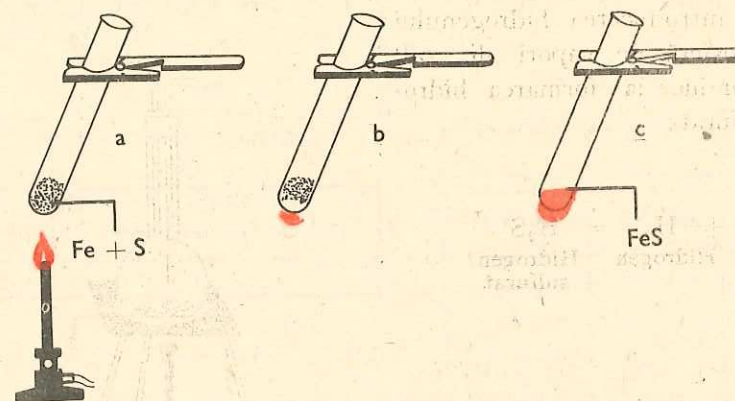
Fig. 3.11. Reacția de formare a sulfurii de fier
