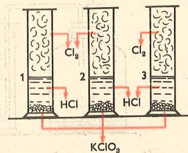
Fig. 2.9. Umplerea a trei cilindri cu clor
