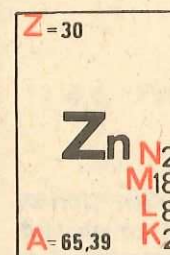
Fig. 11.20. Căsuța zincului în sistemul periodic
