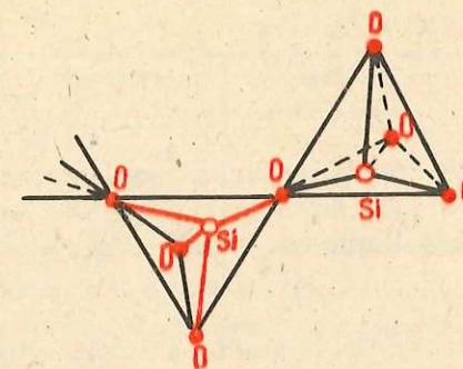
Fig. 5.25. Structura dioxidului de siliciu
