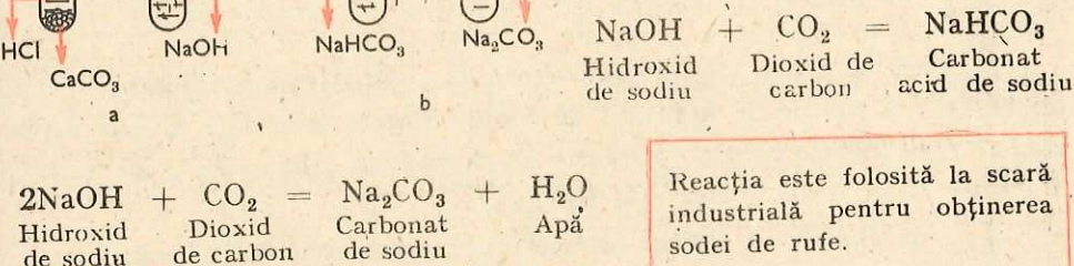
Fig. 7.7. Obținerea carbonaților acid și neutru de sodiu
