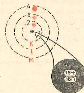
Fig. 3.3. Structura atomului de sulf (Izotopul \frac{32}{16}\text{S} )
