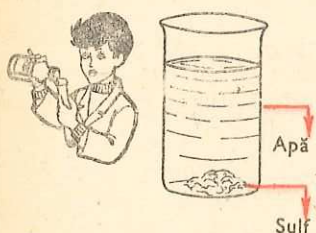
Fig. 3.5. Sulf cristalizat introdus în apă
