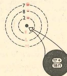
Fig. 2.3. Structura atomului de clor (Izotopul \overset{35}{17}\text{Cl} )
