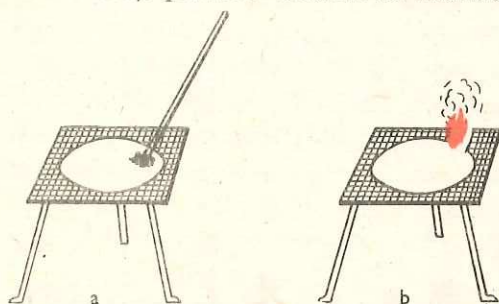
Fig. 11.6. Combinarea fierului cu sulful
