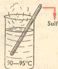
Fig. 3.7. Baston de sulf introdus în apă fierbinte
