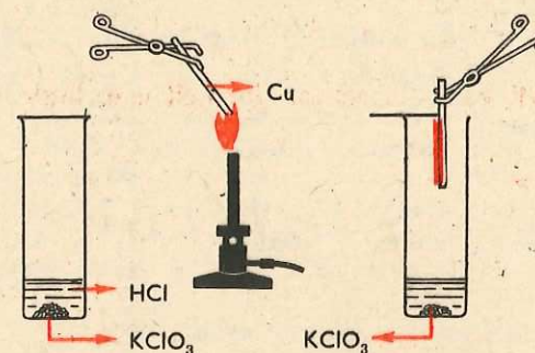
Fig. 6.8, c. Arderea cuprului în clor
