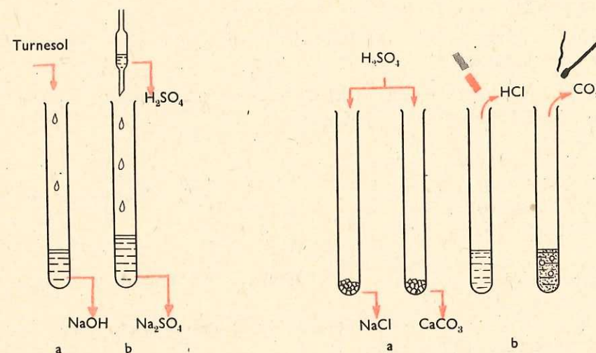
Fig. 3.20. Reacția de neutralizare dintre acidul sulfuric și hidroxidul de sodiu
