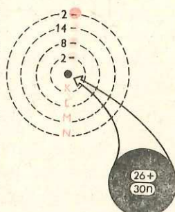
Fig. 11.2. Structura atomului de fier (Izotopul ^{56}_{26}\text{Fe} )
