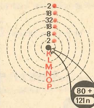
Fig. 11.23. Structura atomului de mercur (Izotopul ^{201}_{80}\text{Hg} )
