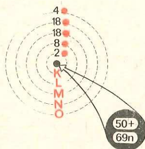
Fig. 10.2. Structura atomului de staniu (Izotopul ^{119}_{50}\text{Sn} )
